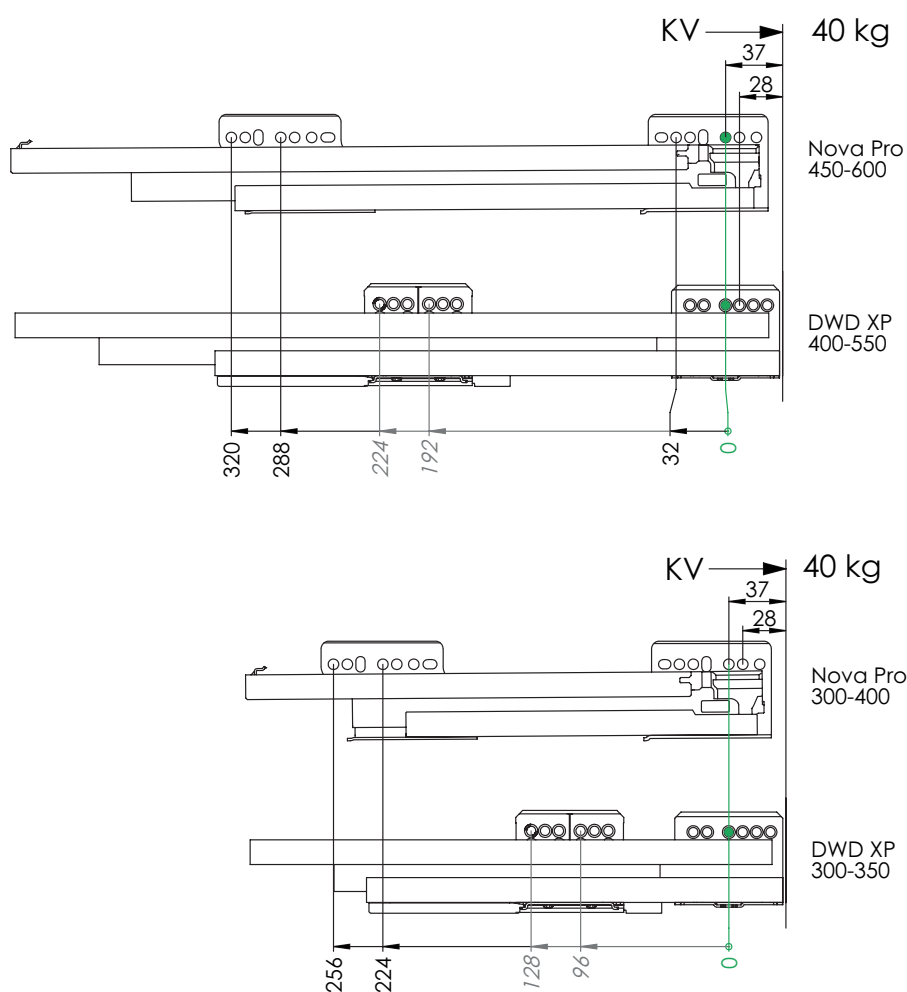
Posiciones de fijación para guía de extracción completa
