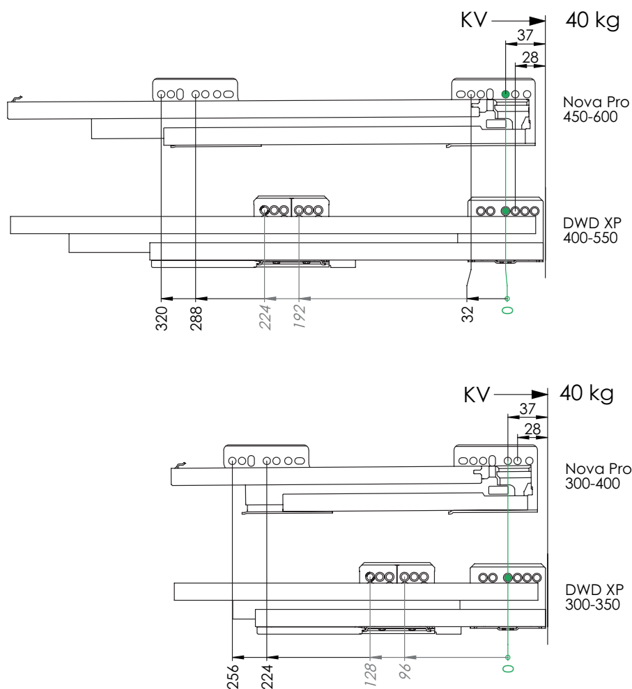
Befestigungspositionen für Vollauszug
