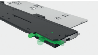
Eine Einheit für alle Anwendungen. Auswurfkraft 3-stufig einstellbar.
