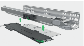
Werkzeuglose Montage und Demontage direkt an der Führung.
