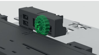
Integrierte, werkzeuglose Tiefenverstellung.
