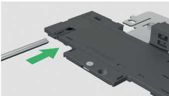
Großer Auslösebereich durch Synchronisationsstange.
