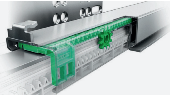
Geringe Öffnungskräfte, exzellente Laufeigenschaften und 100 % Synchronisierung.
